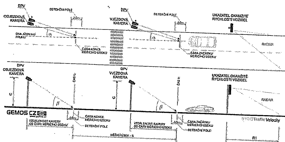
Obr. 1 Uspořádání rychloměru v místě měření
