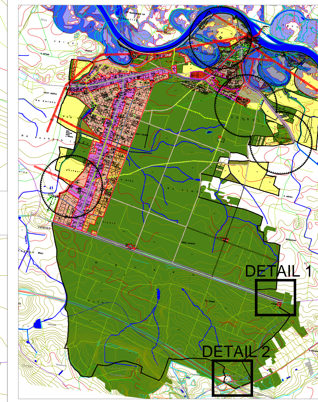
KOORDINAČNÍ VÝKRES 1 : 5000
